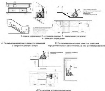
Рисунок 16 – Примеры подъемников различных типов
